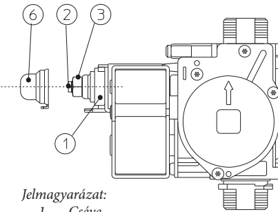
SIT 845 gázszelep
