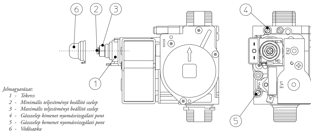
GAS 845 szelep a Nike Mini 28 kazánhoz
